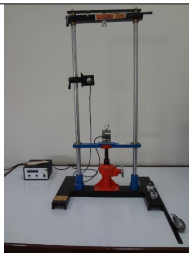
دستگاه تست کمانش
