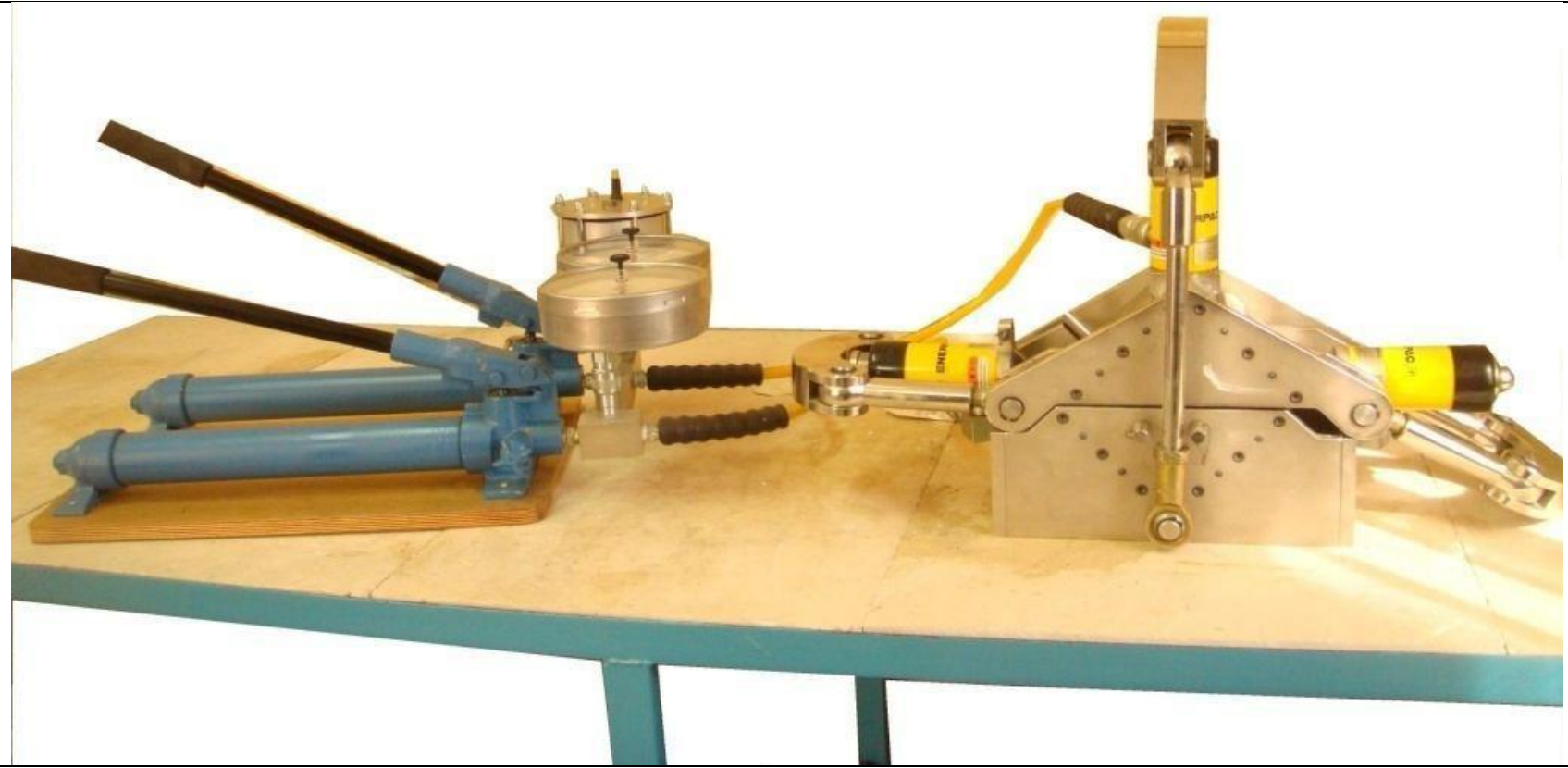
دستگاه آزمایش برش سطوح ضعیف سنگ
